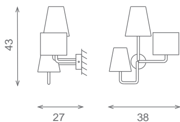
Aplique/Wall lamp Ref.63021 💡3 E14-60w
